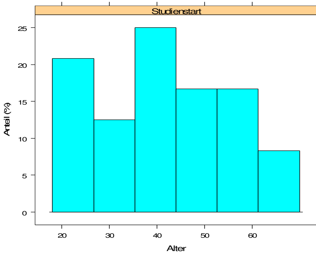
Abbildung 2: Histogramm Alter 2
