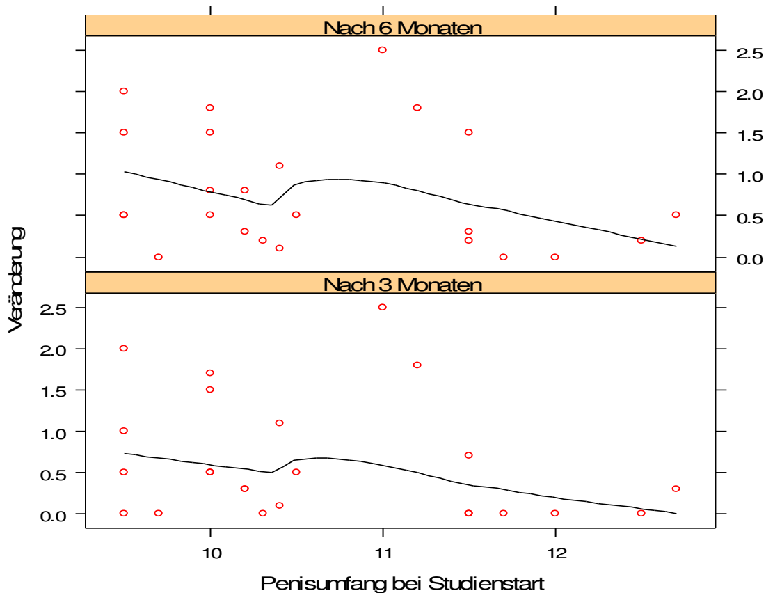
Abbildung 27: Scatterplot Penisumfang 30
