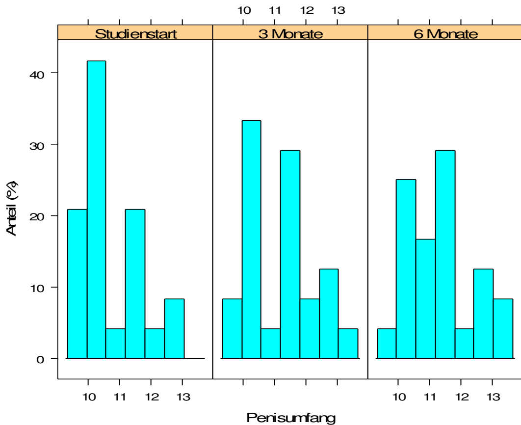
Abbildung 6: Histogramm Penisumfang 6
