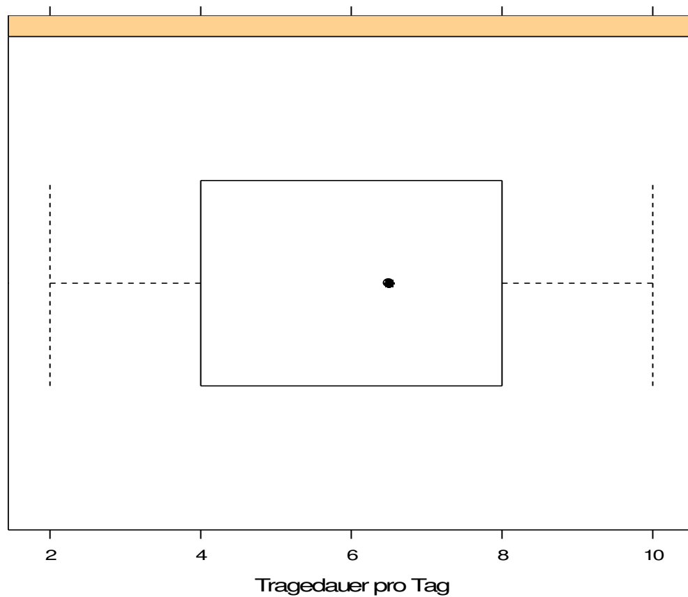
Abbildung 17: Boxplot Tragedauer 17
