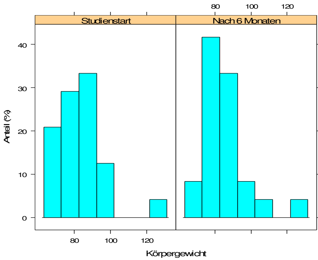
Abbildung 4: Histogramm Körpergewicht 4
