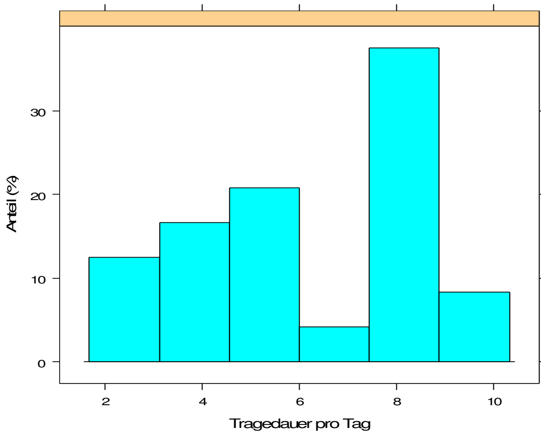
Abbildung 18: Histogramm Tragedauer 18
